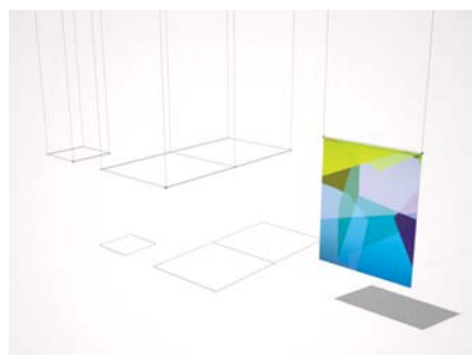
31104 BC rør / BC tube 2,5x2,5 cm. Anvendes til afstivning af bannere og andet ophæng i wirer. Fås i længderne 1m, 2m eller 3m. Kan bære max 15 kg. Used for banners and other decoration hanging from wires. Available in lengths 1m, 2m or 3m. Can carry max 15 kg.
